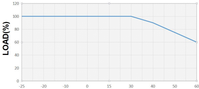
AMBIENT TEMPERATURE(°C)
